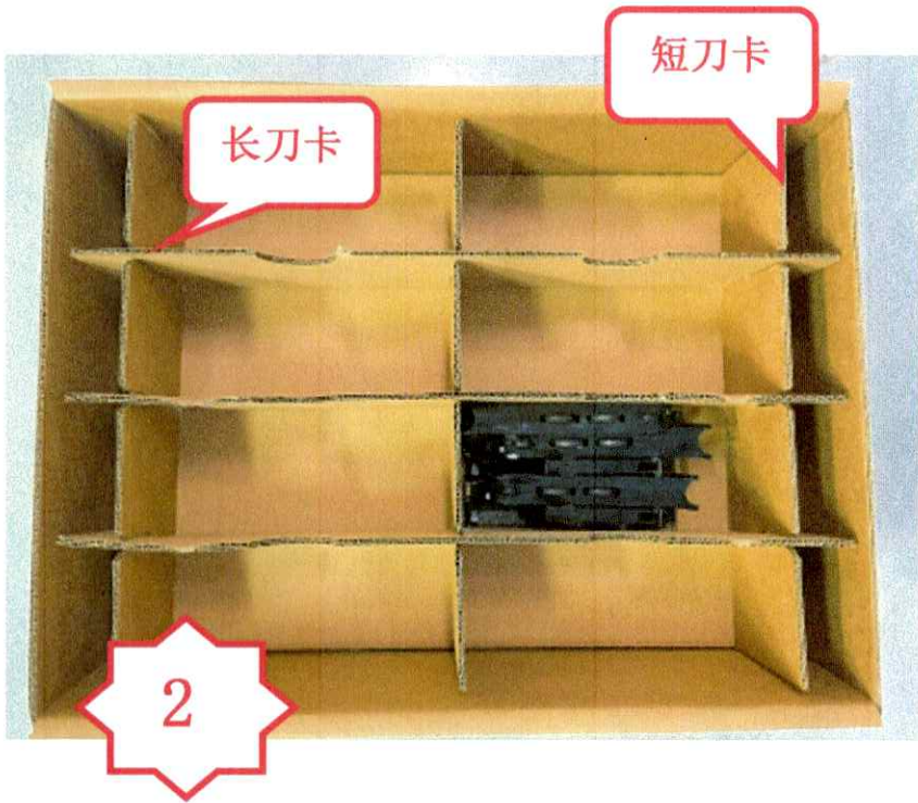
图二，每格放 5 个，每层 8 格 40 个，每箱两层的方式包，共 80 个，同时在底层，顶层各放 1 块隔板。
